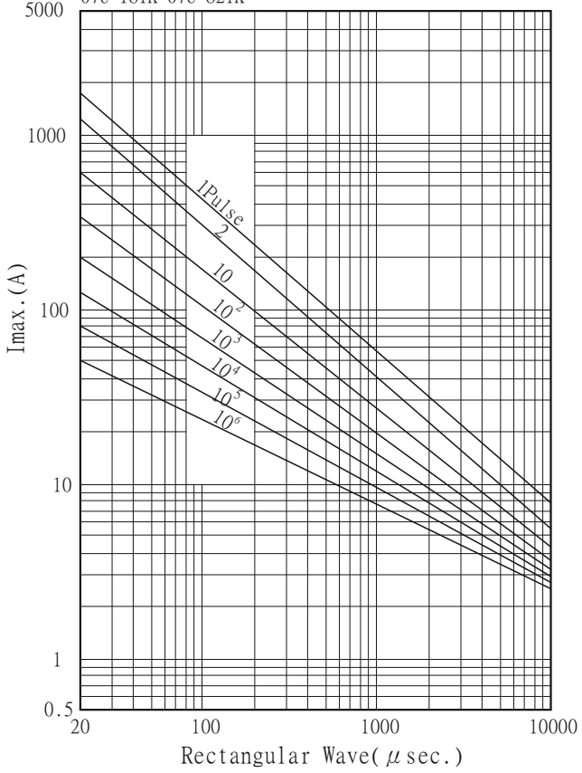
Pulse Life time Ratings - 7mm 07U 181K-07U 821K
