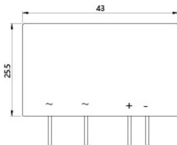
尺寸图
