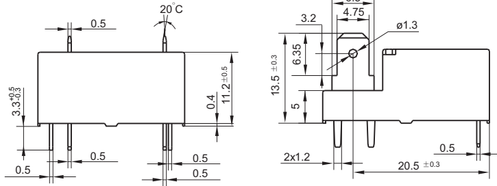
外形图
