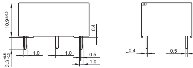
外形图
