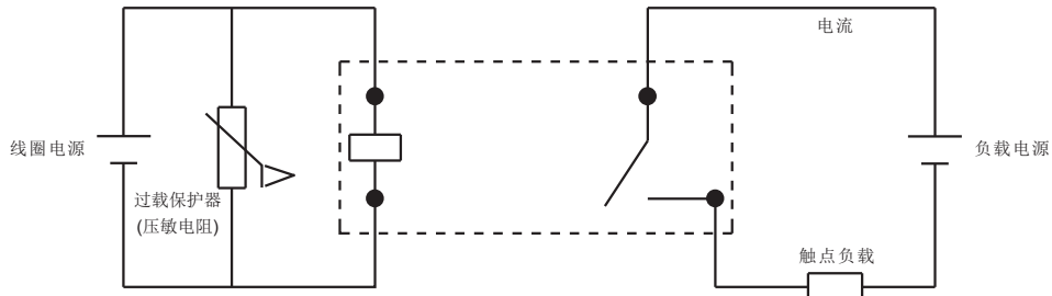
直流负载线路接线图 (底视图)
